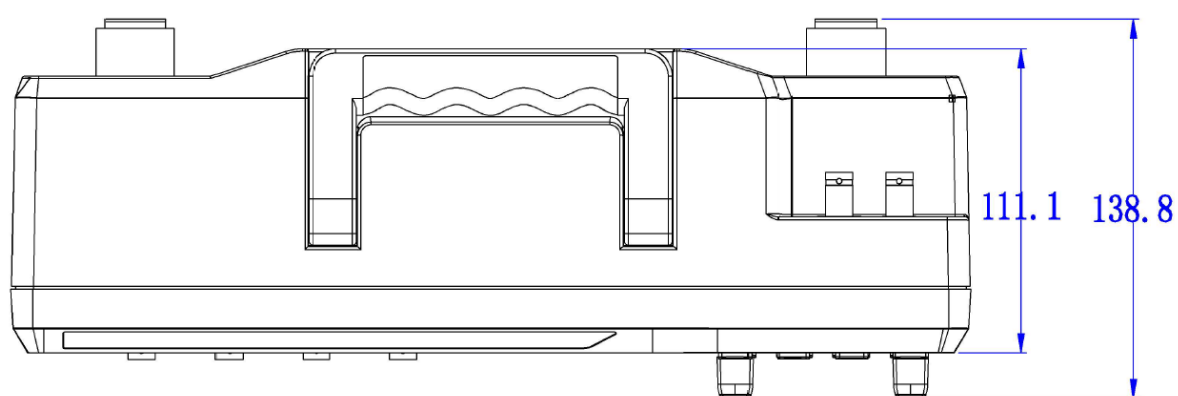
俯视图
